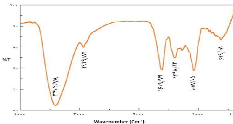
شکل ۳- طیف FT-IR عصاره آبی شکوفه بادام کوهی
