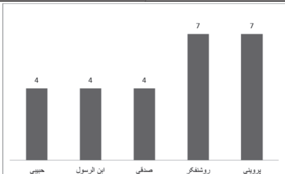
نمودار شماره (۶) - پرتولیدترین نویسندگان
